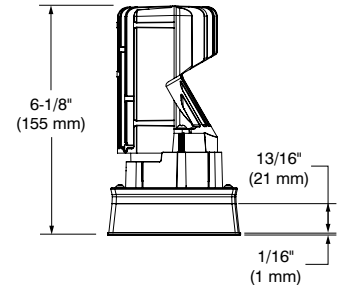
FLANGELESS TRIM
