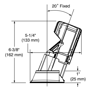
FLANGELESS TRIM
